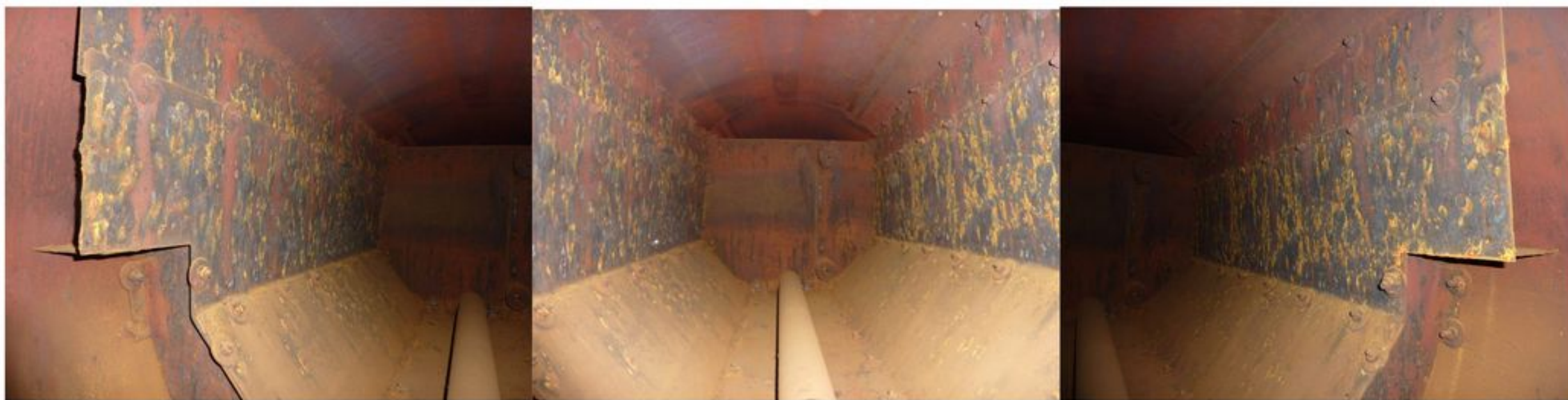
Внутренняя поверхность барабана парового котла ДЕ 25-14 («соленый» отсек) до отмывки и консервации
